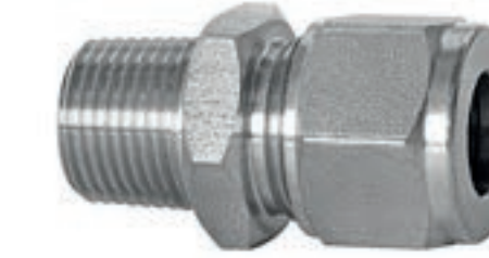
303 kalite 1/4" boru için 3/8" NPT erkek bağlantı
