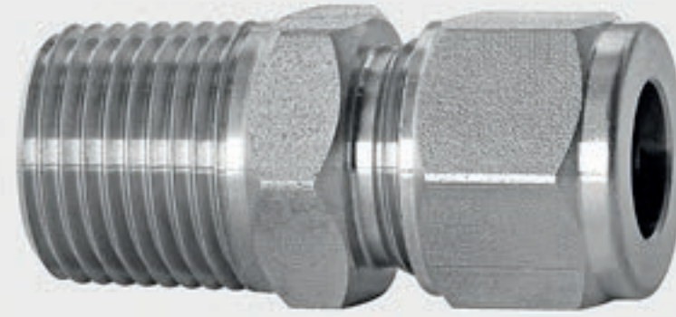
303 kalite 12 mm boru için 1/2" NPT erkek bağlantı
