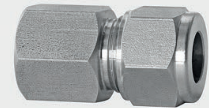
303 kalite 12 mm boru için 3/8" NPT dişi bağlantı
