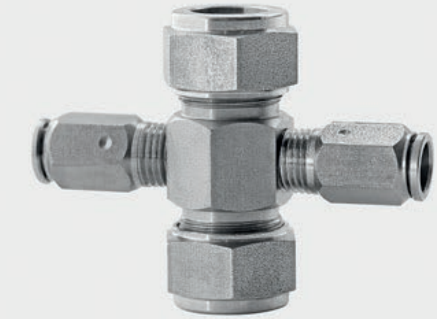
303 kalite 1/4" borudan 1/4" NORMATIC® boruya X bağlantı
