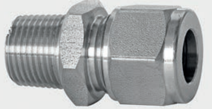
303 kalite 12 mm boru için 3/8" NPT erkek bağlantı
