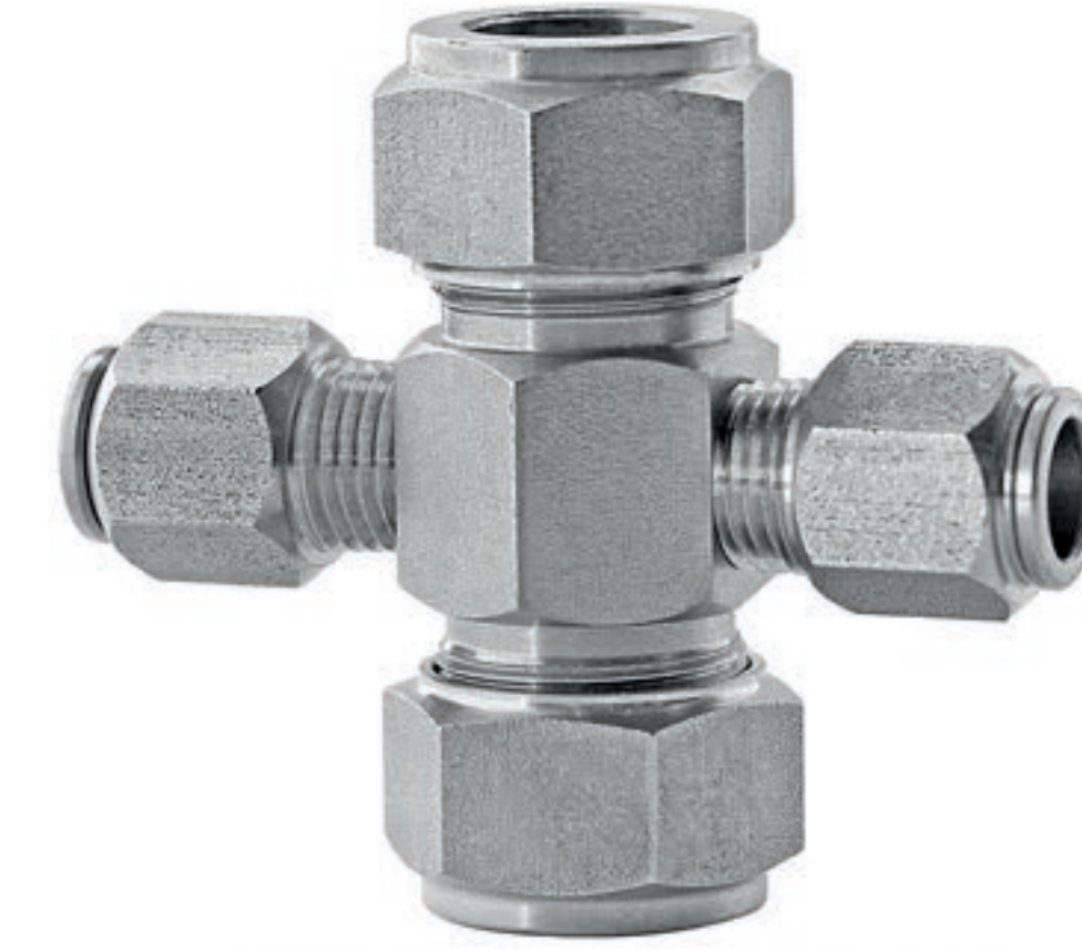
303 kalite 12 mm borudan 3/8" nylon boruya X bağlantı
