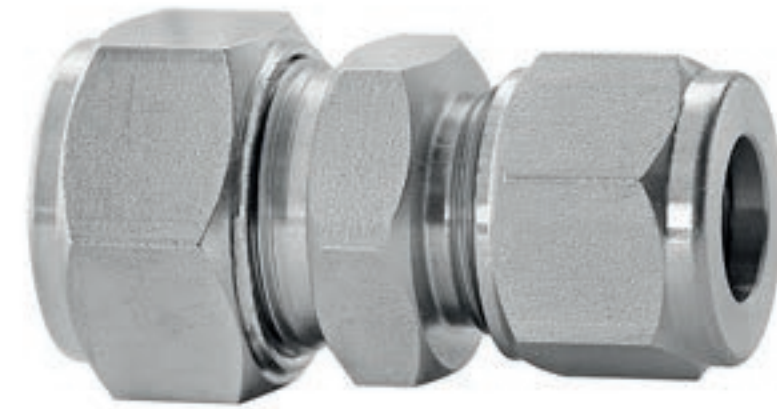
303 kalite 16 mm borudan 12 mm boruya redüksiyon
