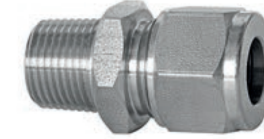
303 kalite 3/8" boru için 3/8" NPT erkek bağlantı
