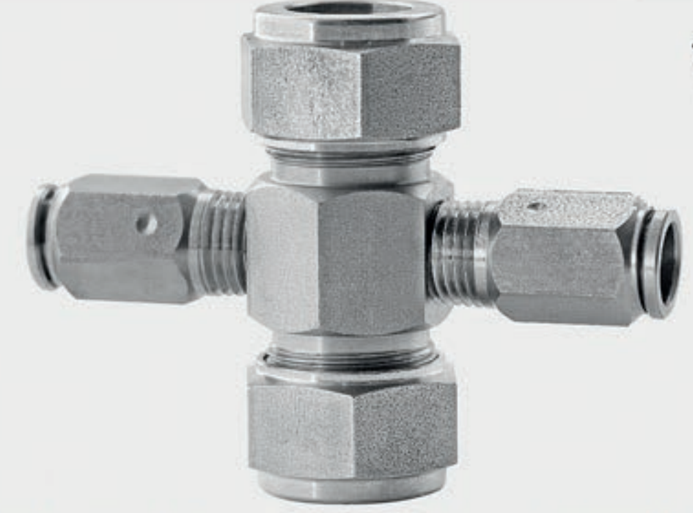
303 kalite 12 mm borudan 10 mm NORMATIC® boruya X bağlantı
