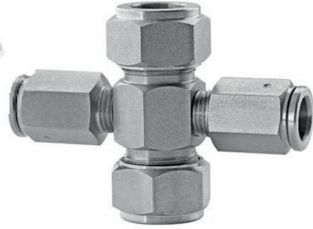
303 kalite 1/2" borudan 3/8" NORMATIC® boruya X bağlantı
