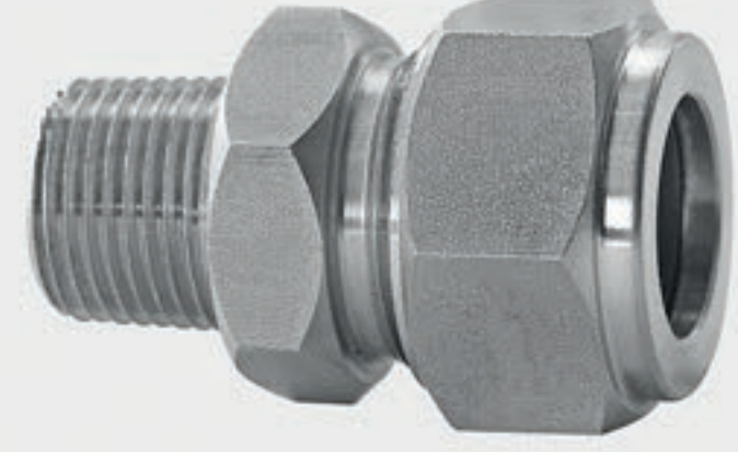
303 kalite 16 mm boru için 3/8" NPT erkek bağlantı
