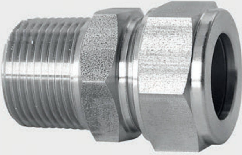
303 kalite 20 mm boru için 3/4" erkek bağlantı
