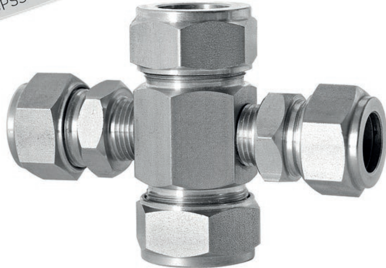
303 kalite 20 mm borudan 16 mm boruya X bağlantı
