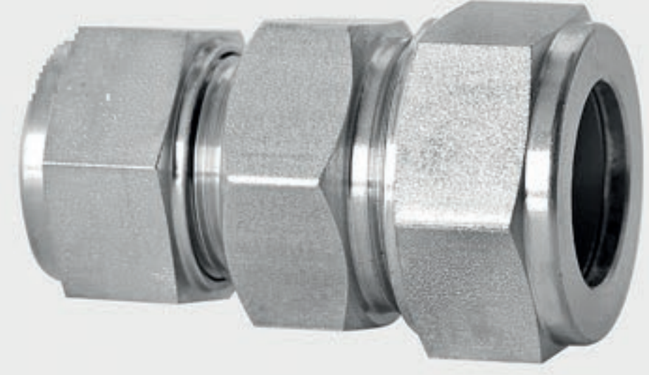
303 kalite 20 mm borudan 16 mm boruya redüksiyon
