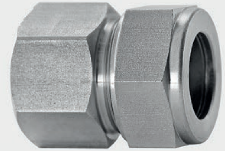
303 kalite 20 mm boru için 3/8" NPT dişi bağlantı
