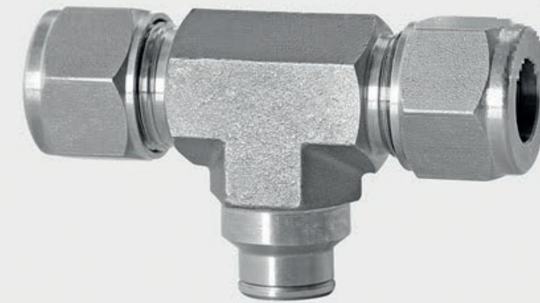
303 kalite 12 mm borudan 10 mm NORMATIC® boruya T bağlantı ( 12 mm - 3/8" - 12 mm )
