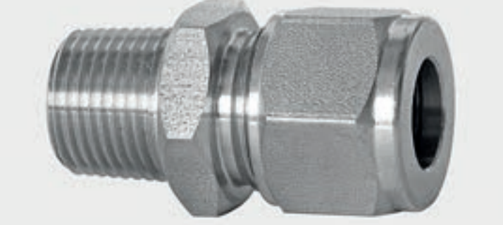
303 kalite 1/2" boru için 3/8" NPT erkek bağlantı
