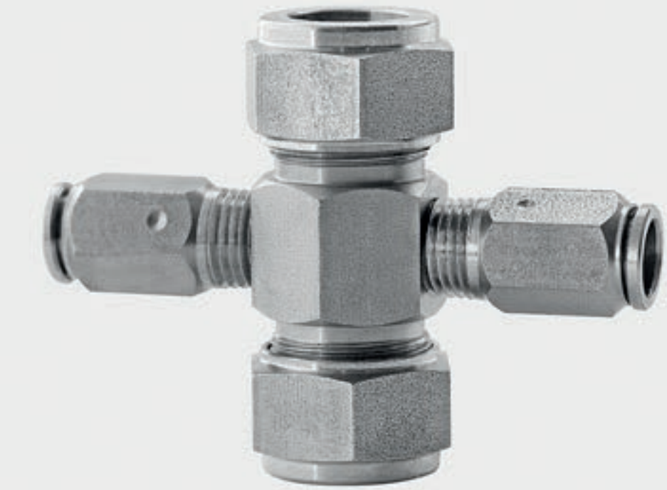
303 kalite 3/8" borudan 1/4" NORMATIC® boruya X bağlantı
