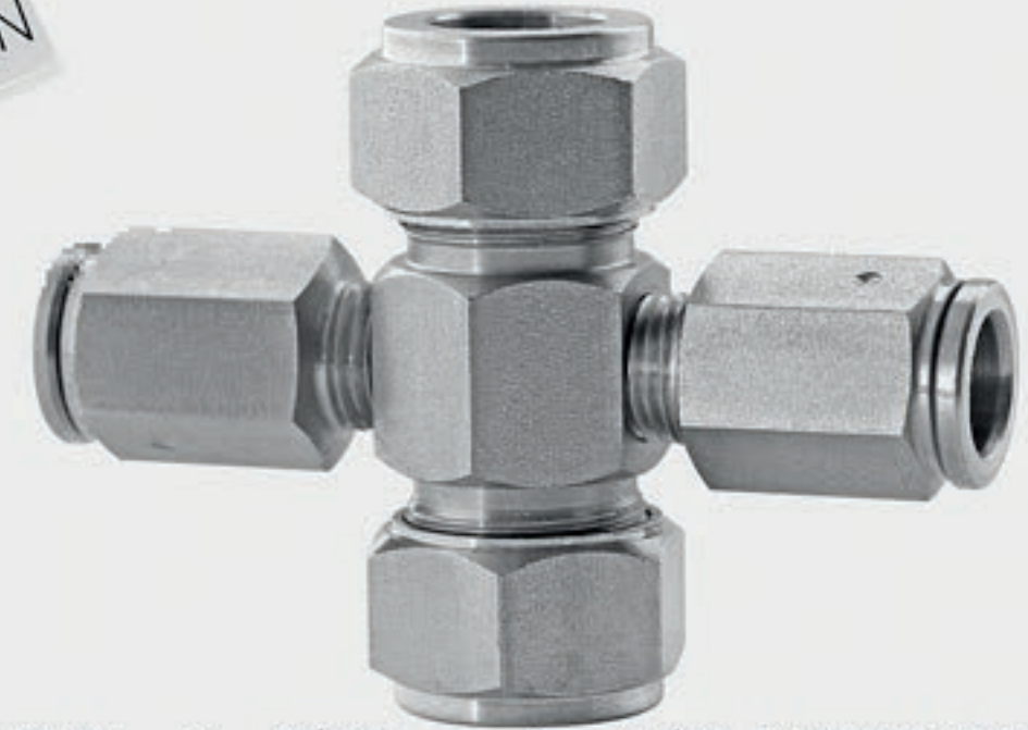
303 kalite 3/8" borudan 3/8" NORMATIC® boruya X bağlantı
