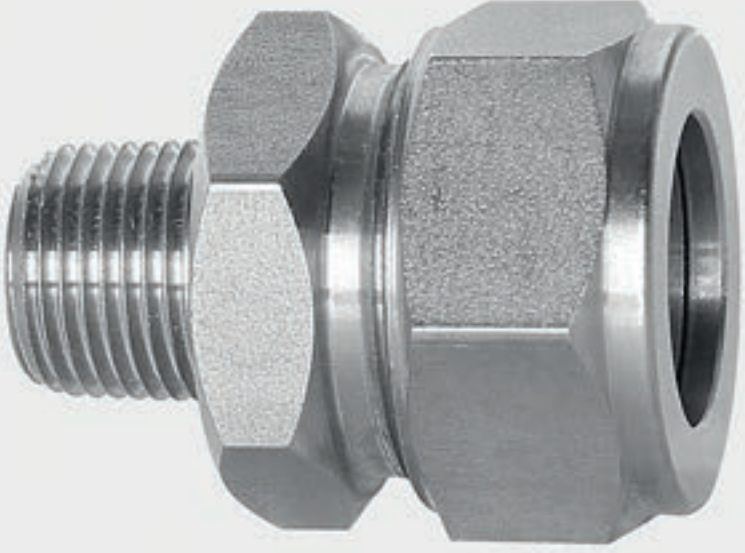
303 kalite 20 mm boru için 3/8" NPT erkek bağlantı
