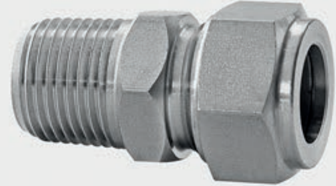
303 kalite 16 mm boru için 1/2" NPT erkek bağlantı
