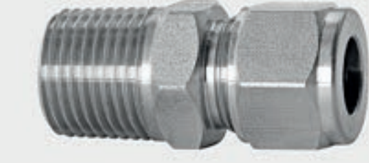
303 kalite 1/4" boru için 1/2" NPT erkek bağlantı
