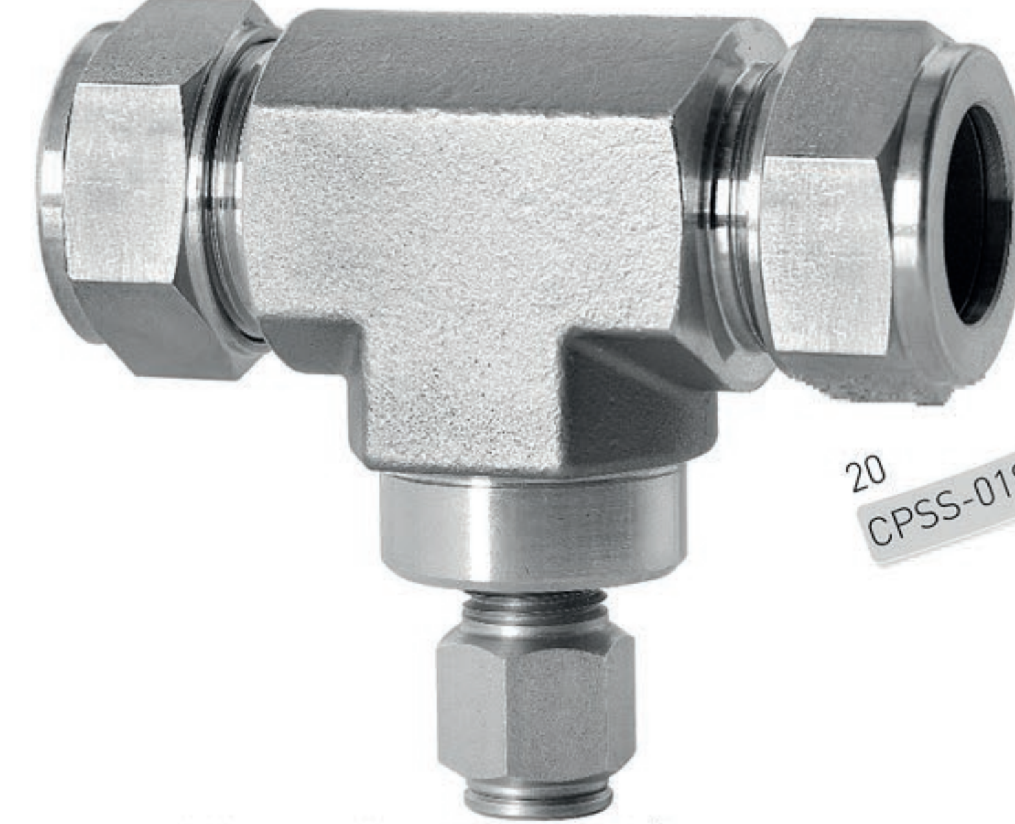
303 kalite 20 mm borudan 3/8" nylon boruya T bağlantı
