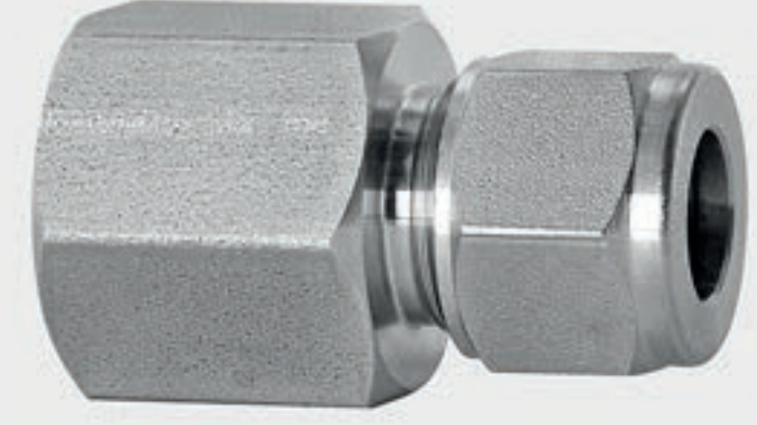
303 kalite 12 mm boru için 1/2" NPT dişi bağlantı
