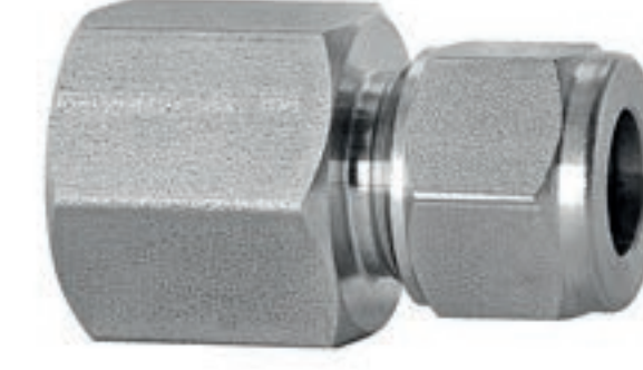
303 kalite 3/8" boru için 1/2" NPT dişi bağlantı
