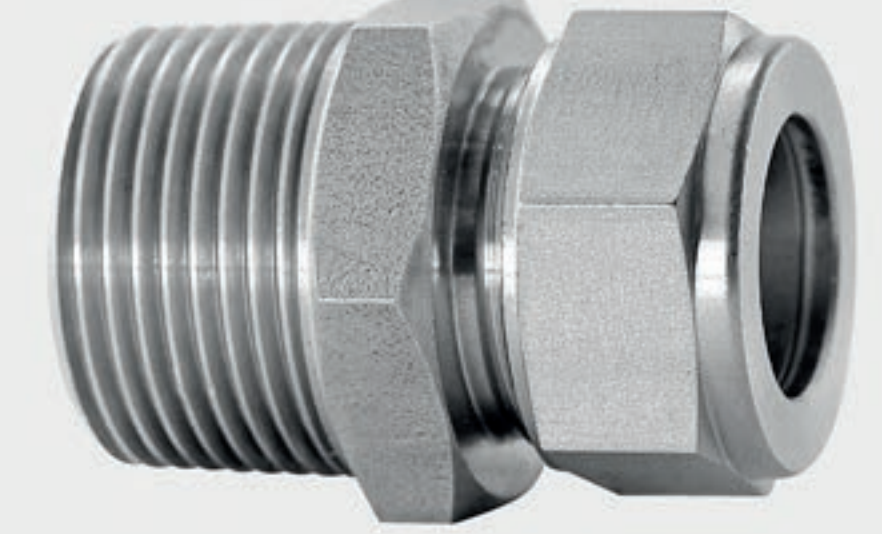
303 kalite 20 mm boru için 1" NPT erkek bağlantı
