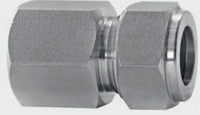
303 kalite 16 mm boru için 1/2" NPT dişi bağlantı
