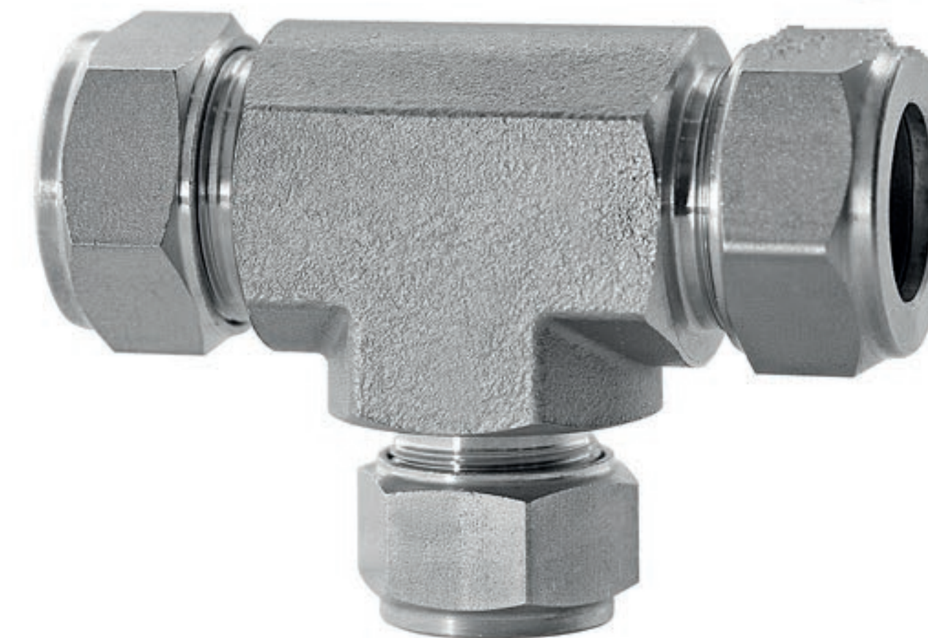
303 kalite 20 mm borudan 16 mm boruya T bağlantı ( 20-16-20 )
