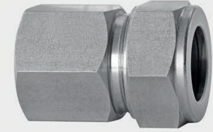
303 kalite 20 mm boru için 1/2" NPT dişi bağlantı
